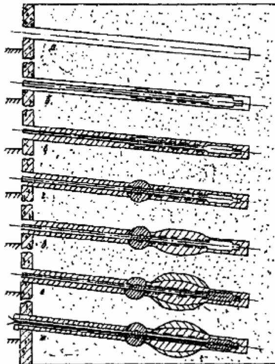
Черт. 4. Технологическая последовательность устройства постоянного анкера с манжетной трубой при внутреннем расположении тяги из канатной арматуры
