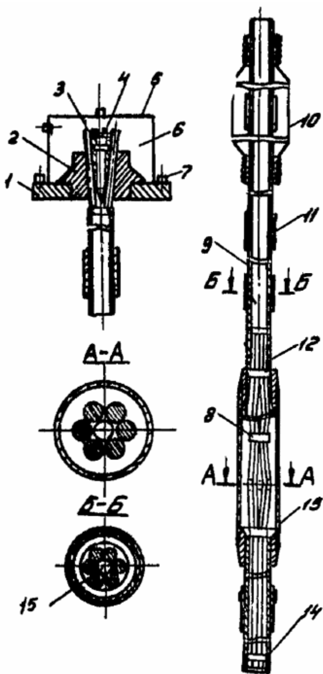
Черт. 3. Постоянный инъекционный анкер с манжетной трубой при внутреннем расположении анкерной тяги из канатной арматуры
